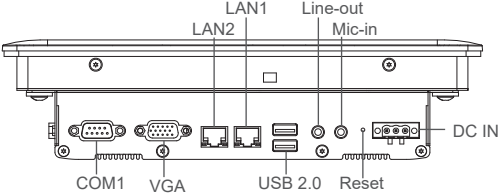
Right I/O
