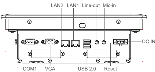
Right I/O
