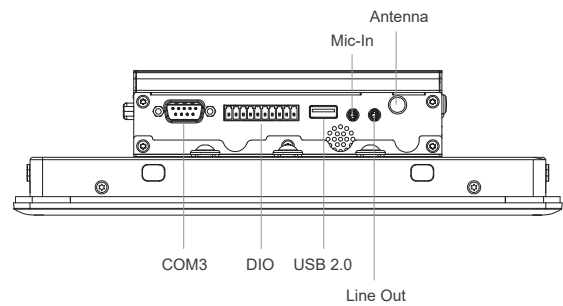
Right I/O
