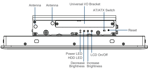
Left I/O
