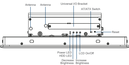
Left I/O
