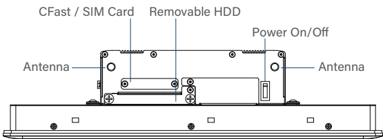
Left I/O
