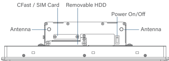
Left I/O
