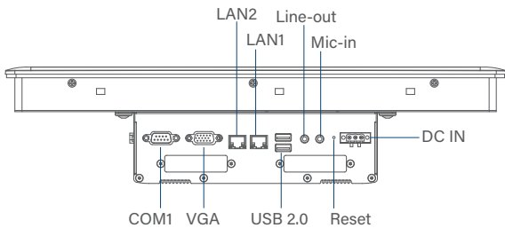
Right I/O
