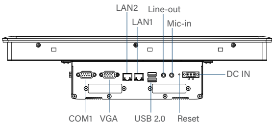
Right I/O
