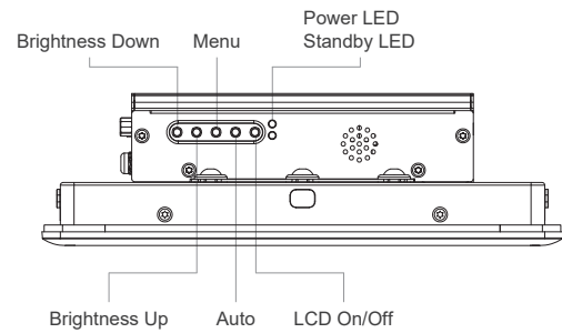
Right I/O
