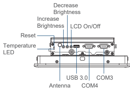
Left I/O
