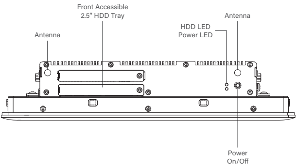
Left I/O
