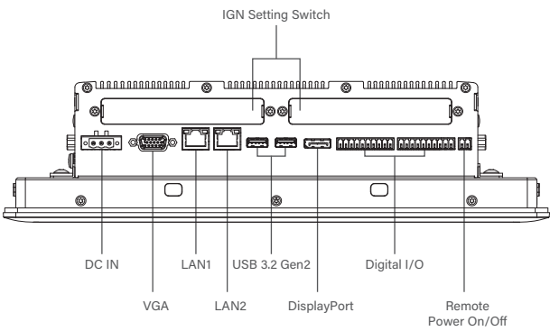
Right I/O
